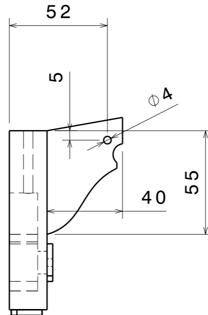
Vue de gauche Echelle : 1:2
