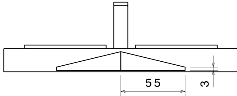
Vue de dessous Echelle : 1:2
