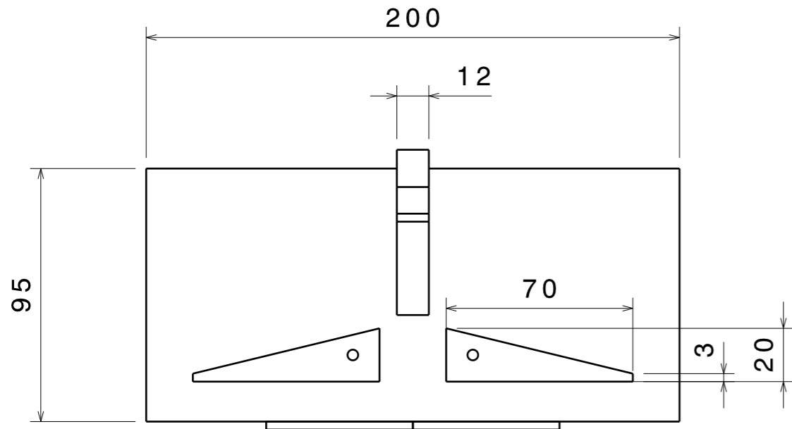
Vue de face Echelle : 1:2
